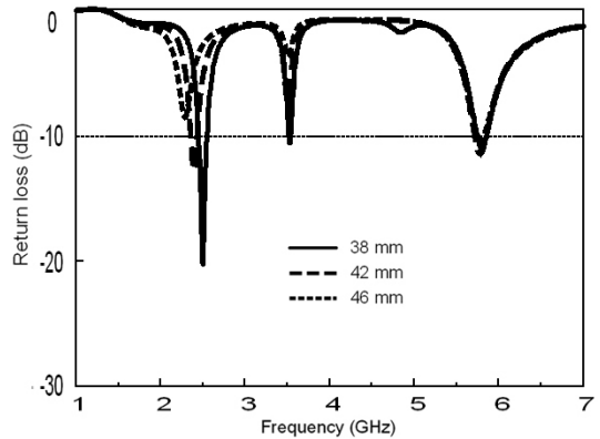
그림 3. 큰 E 형태의 세로 길이 l_1 의 변화에 따른 반사 손실 Fig. 3. Variation of return loss with respect to the vertical length of large E-shaped.
