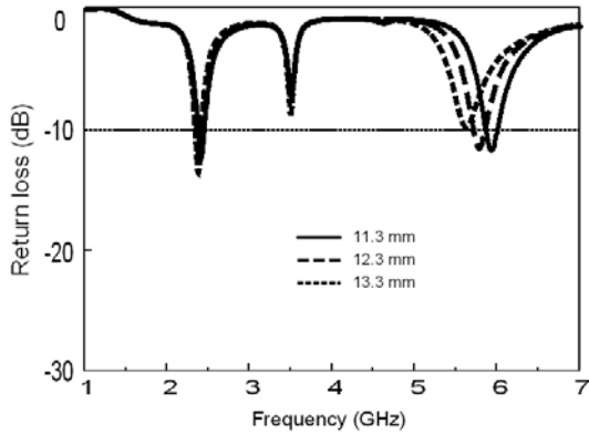
그림 4. 작은 E 형태의 세로 길이 l_2 의 변화에 따른 반사 손실
