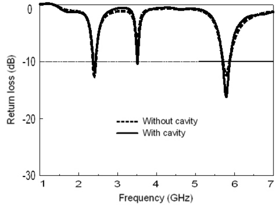
그림 2. 안테나의 반사 손실 Fig. 2. Return loss of the simulated antenna.
