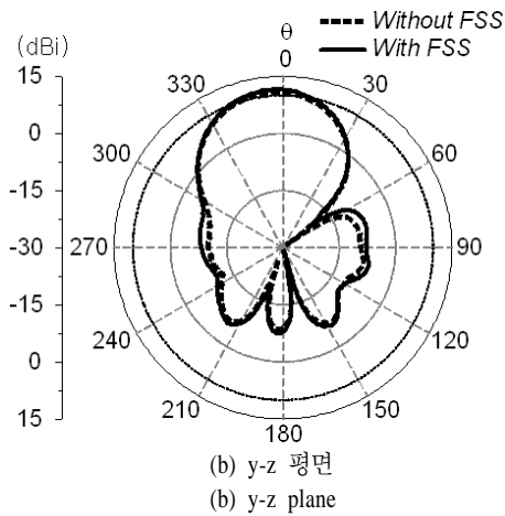
그림 17. 2.46 GHz에서의 복사 패턴 Fig. 17. Radiation patterns at 2.46 GHz.
